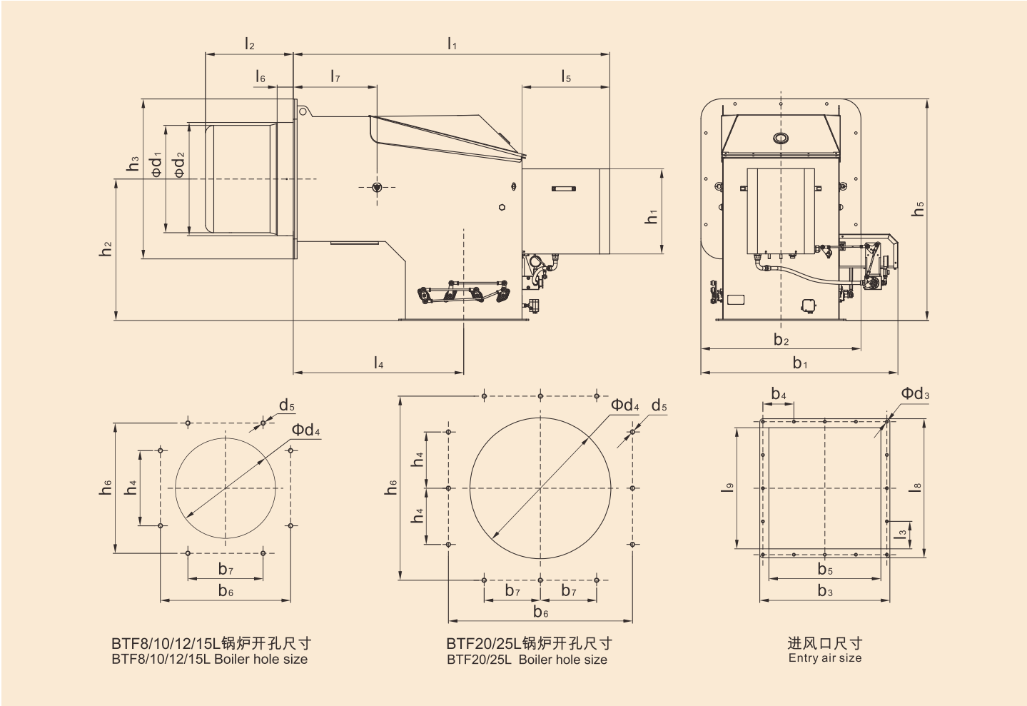
外形尺寸图 Outline size diagram 型号Model: BTF8L...25L
